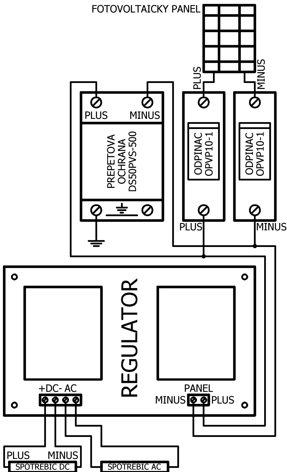
Doporučené schéma zapojení pro 1. a 2. režim činnosti
