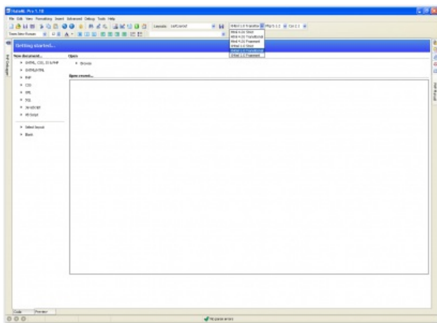
HateML Pro
